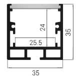
LCP3535 (Pendant)
